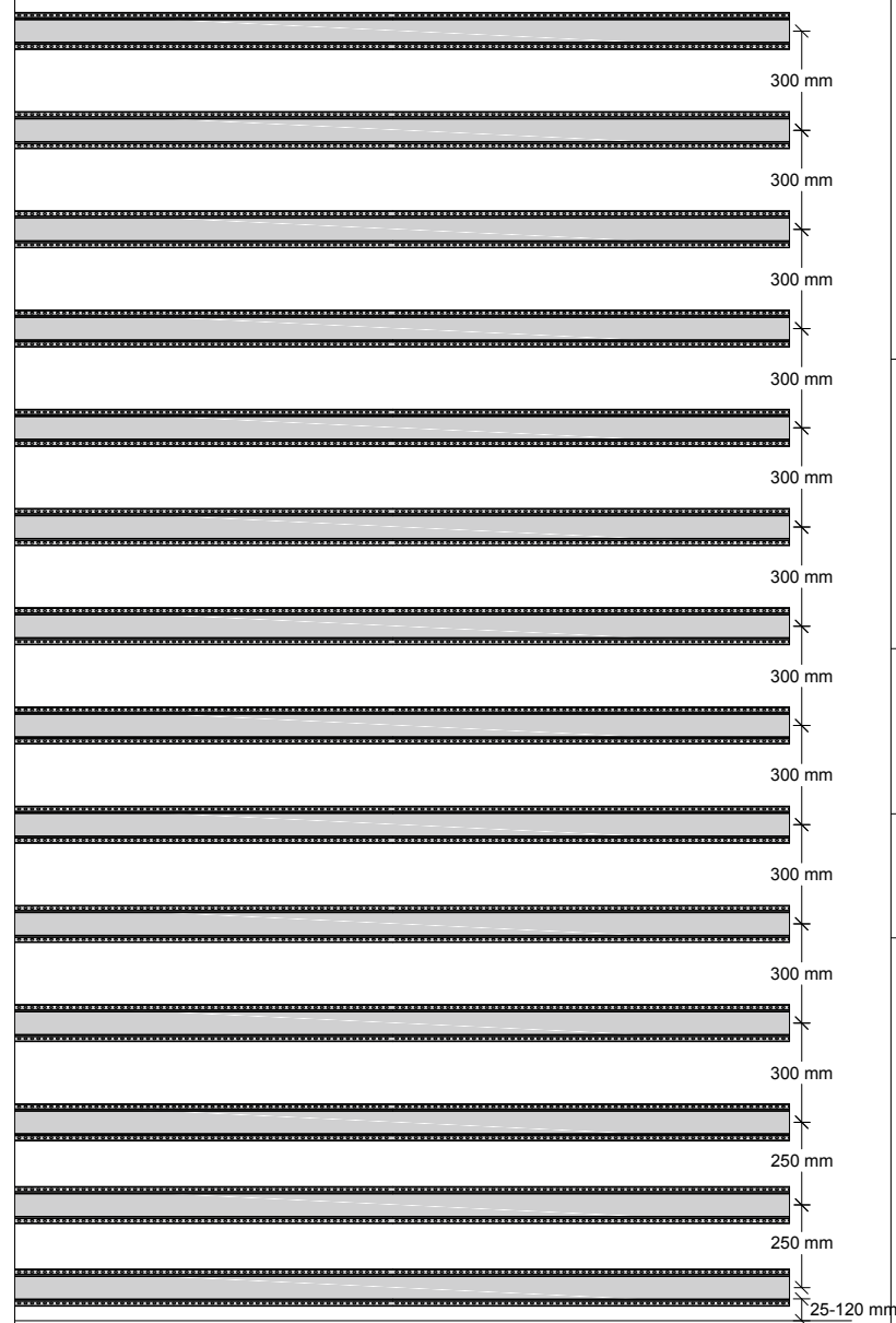
VFL STÅLPROFIL 70/25 CC 300MM
